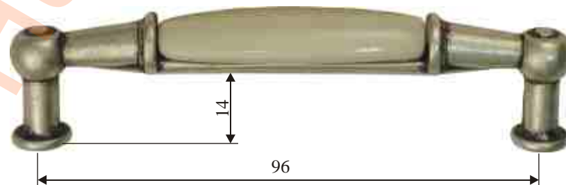
9029/Av altverzinkt mit altweißem Porzellan
